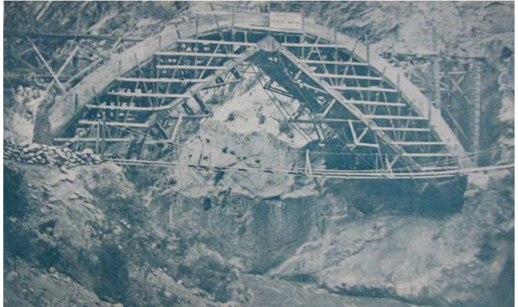
Figura 11: El puente principal del camino a Cacheuta, durante su construcción.
